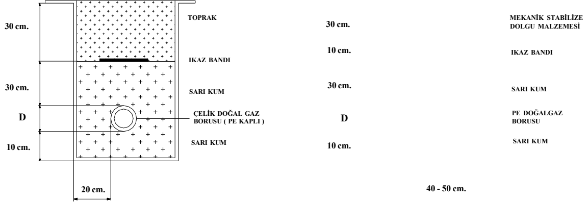
Şekil 2 - Toprakaltı hat detayı (PE boru)
