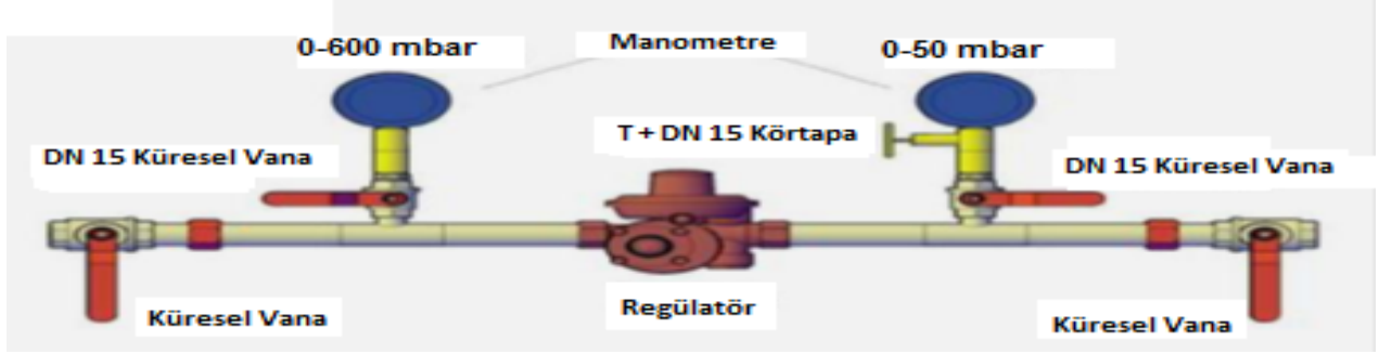
Şekil 13 – Regülatör Bağlantısı
