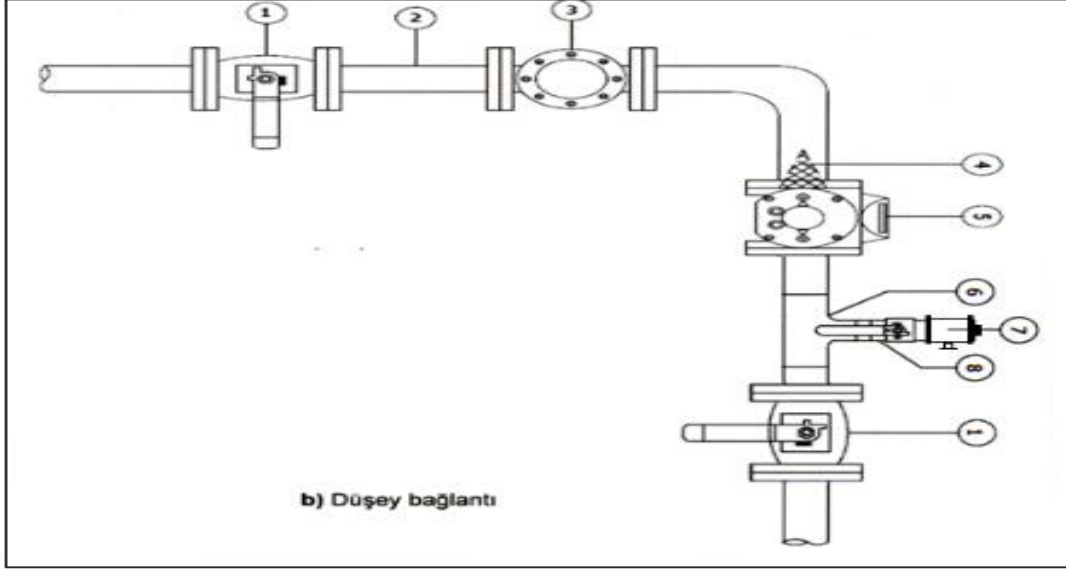
Şekil 11 - Rotary sayaçlara ait bağlantı detayı
