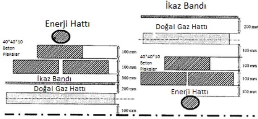
Şekil 4 – Doğalgaz hattı ile elektrik kabloları arasındaki mesafe
