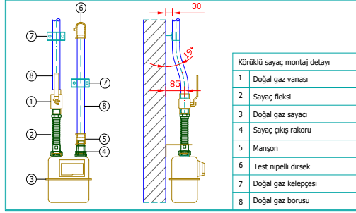
Şekil 10 - Sayaç Bağlantısı Detayı Örneği
